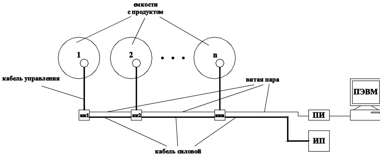
Рис. 2. Построение уровнемера.
