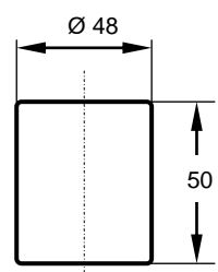
Поплавок Тип II
