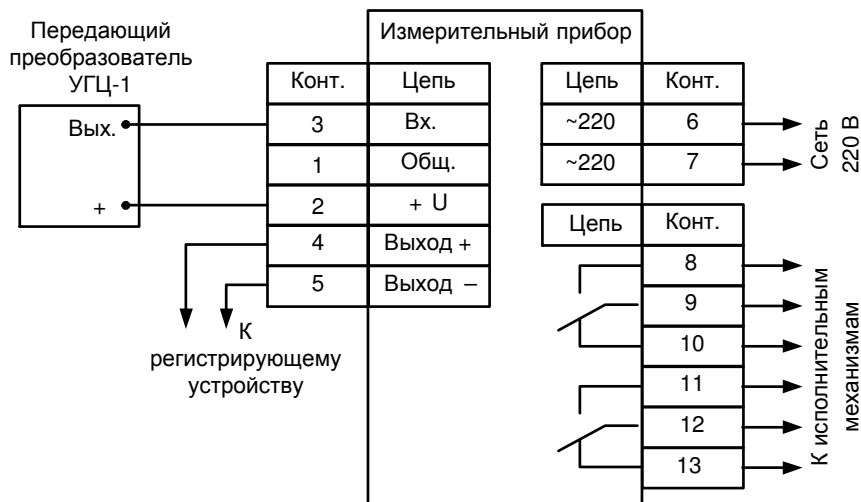
а) внешние соединения для обычного исполнения
