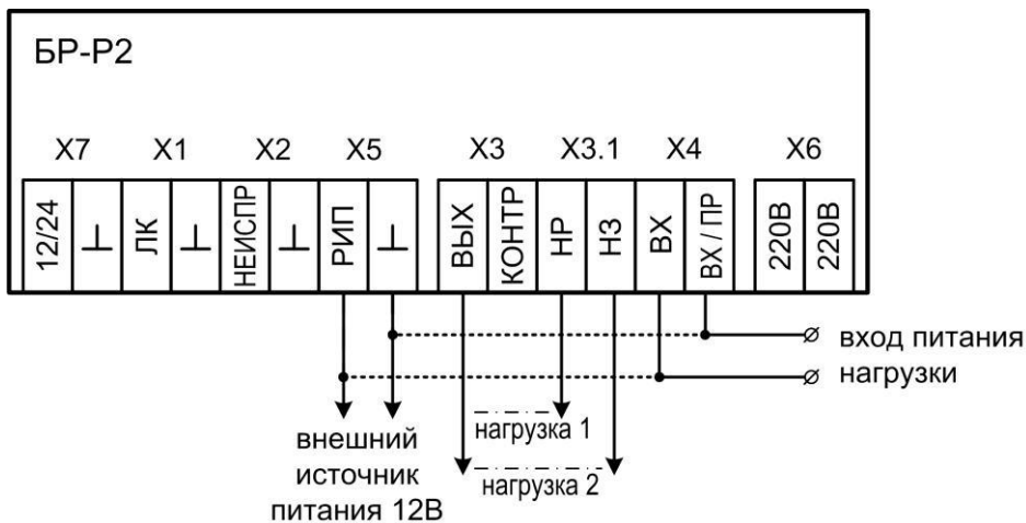
Рис.В9 Универсальная переключающая схема подключения. Питание БР-Р2 от РИП 12В. Пунктиром показан вариант питания нагрузки от входа РИП БР-Р2
