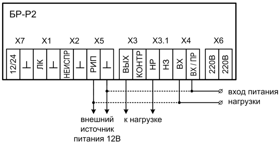
Рис.В6 Универсальная замыкающая схема подключения. Питание БР-Р2 от РИП 12В. Пунктиром показан вариант питания нагрузки от входа РИП БР-Р2
