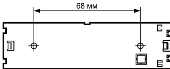
Рис.14в Основание Термо-P2. Присоединительные размеры
