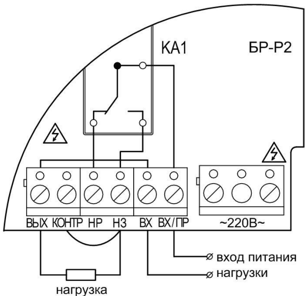
Рис.В15 Схема подключений БР-Р2 при контроле исполнительной линии «H3» - «ВЫХ». БР-Р2 в состоянии Выключено
