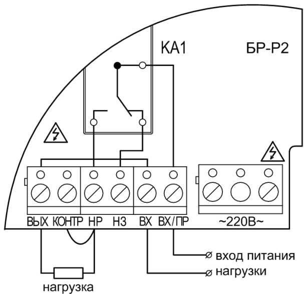
Рис.В14 Схема подключений БР-Р2 при контроле исполнительной линии «HP» - «ВЫХ». БР-Р2 в состоянии Выключено
