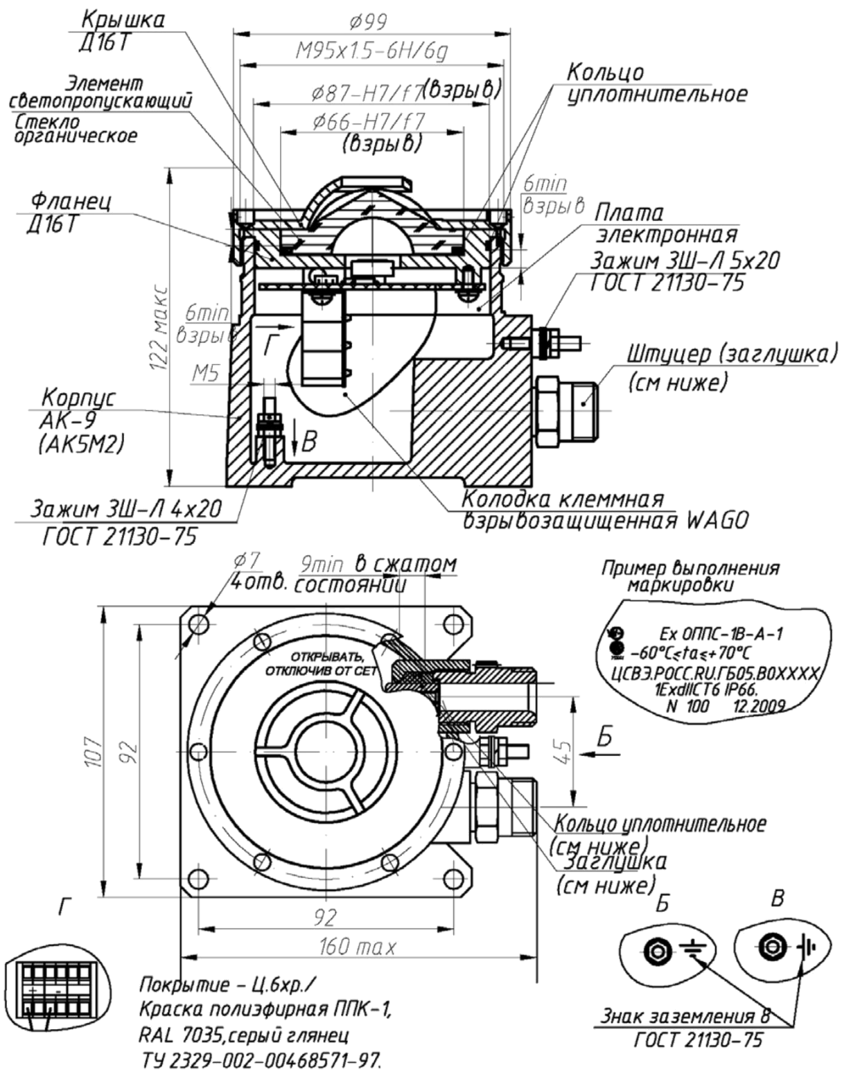
Рис. А.2 Габаритный чертёж световых Оповещателей ExOΠΠC-1B-A, ExOΠΠC-1B-P-A, ExOΠΠC-1B-A-18 в алюминиевом корпусе, совмещённый с чертежом взрывозащиты
