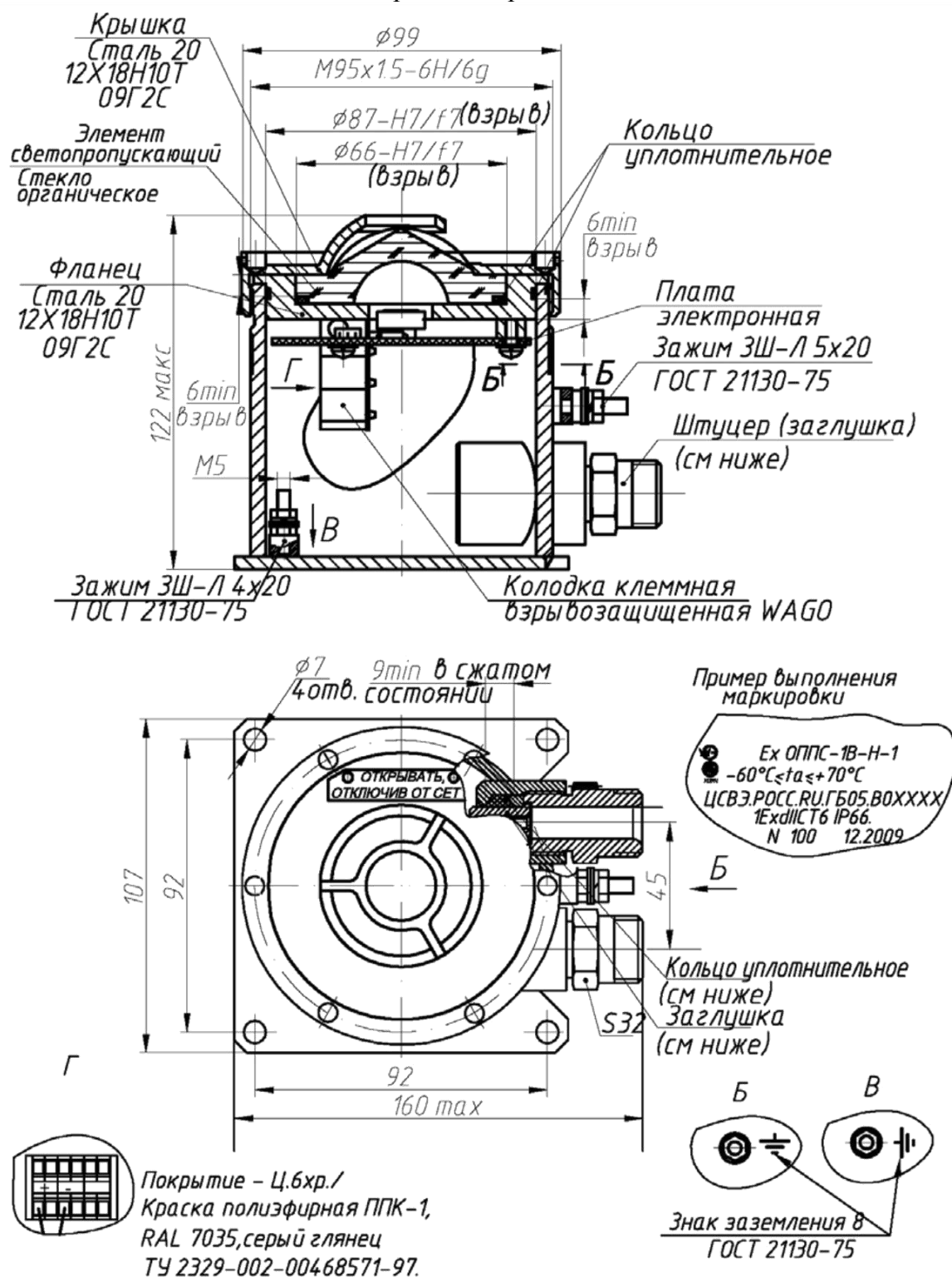
Рис. А.1 Габаритный чертёж световых Оповещателей ExOPLS-1B-H, ExOPLS-1B-P-H, ExOPLS-1B-H-18, ExOPLS-1B-C, ExOPLS-1B-P-C, ExOPLS-1B-C-18 в сталь-ном корпусе, совмещённый с чертежом взрывозащиты
