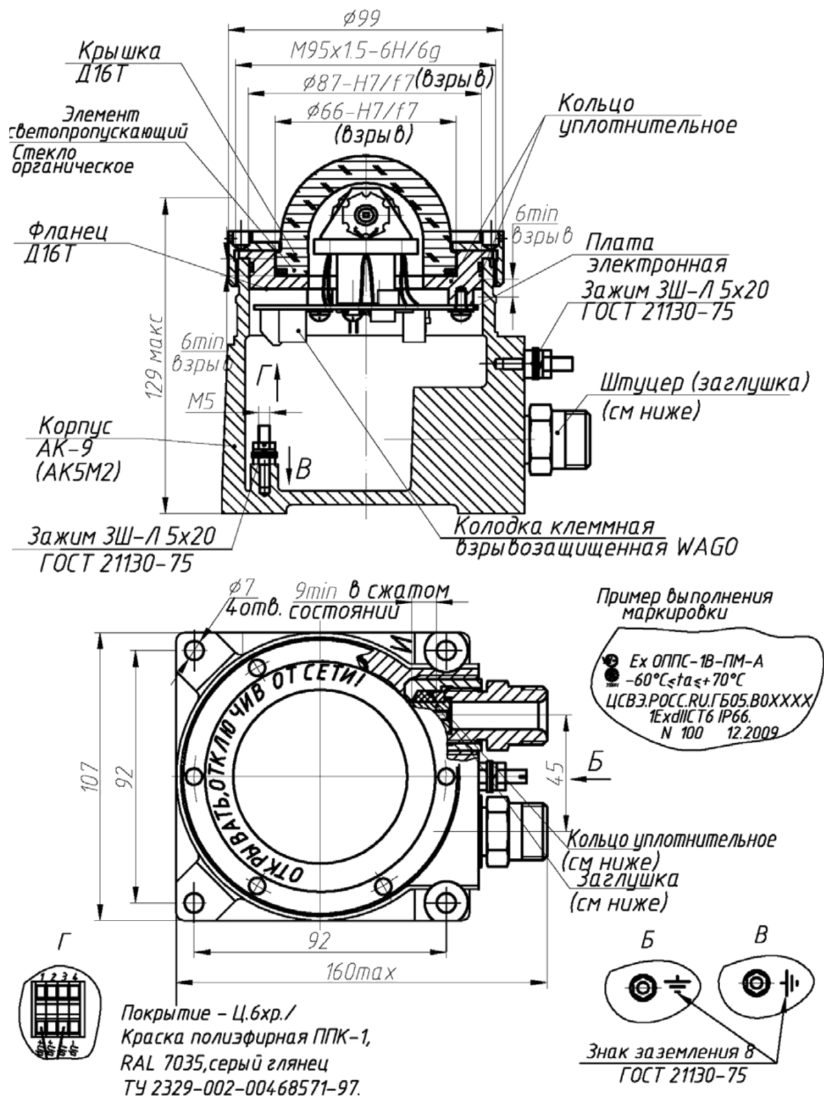
Рис. А.4 Габаритный чертёж световых Оповещателей повышенной мощности ExОППС- 1В-ПМ-А, ExОППС-1В-ПМ-А-18 в алюминиевом корпусе, совмещённый с чертежом взрывозащиты
