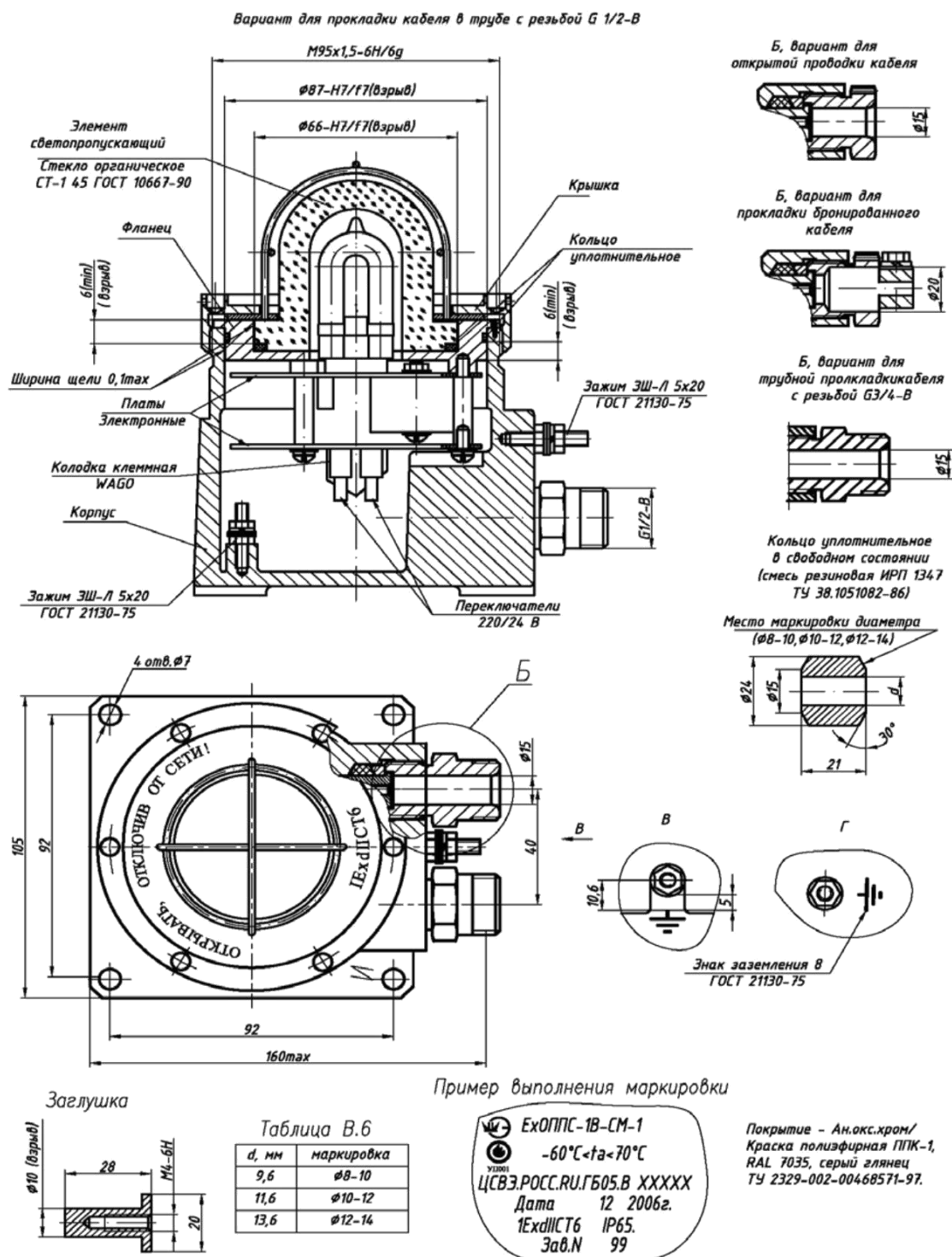
Рис. А.9 Габаритный чертёж светового Оповещателя ExOPPC-1B-CM в алюминиевом корпусе, совмещённый с чертежом взрывозщиты
