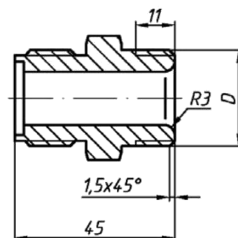
Рис. 3 Остальное – см. рис. 1 Штуцер для прокладки бронированного кабеля (планки 908.2013.00.016, винты М5 и гайки М5 условно не показаны)
