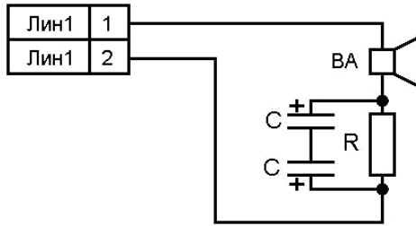
Рис. 3 Схема электрическая «АС-2-1» ВА – головка громкоговорителя динамическая, номинальное электрическое сопротивление – 4 Ом; C=470 мкФ, 16 В; R=10 Ом, 0,25 Вт
