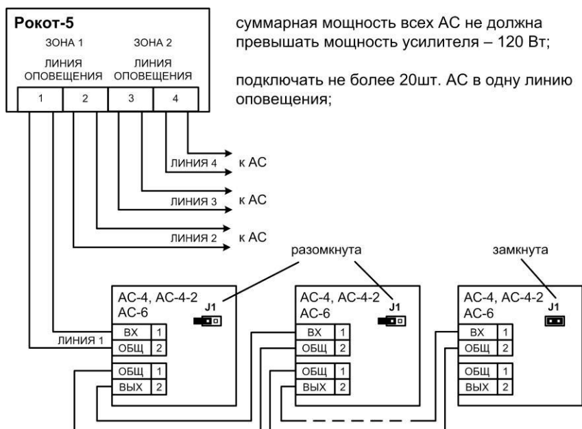
Рис.4а Схема подключений AC-4, AC-4-2, AC-6 к линиям оповещения
