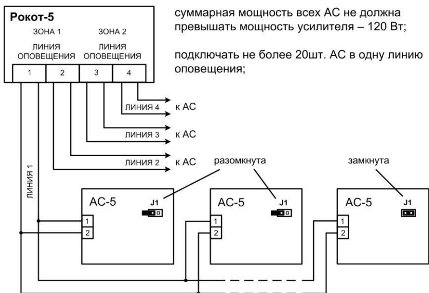
Рис.4б Схема подключений AC-5 к линиям оповещения
