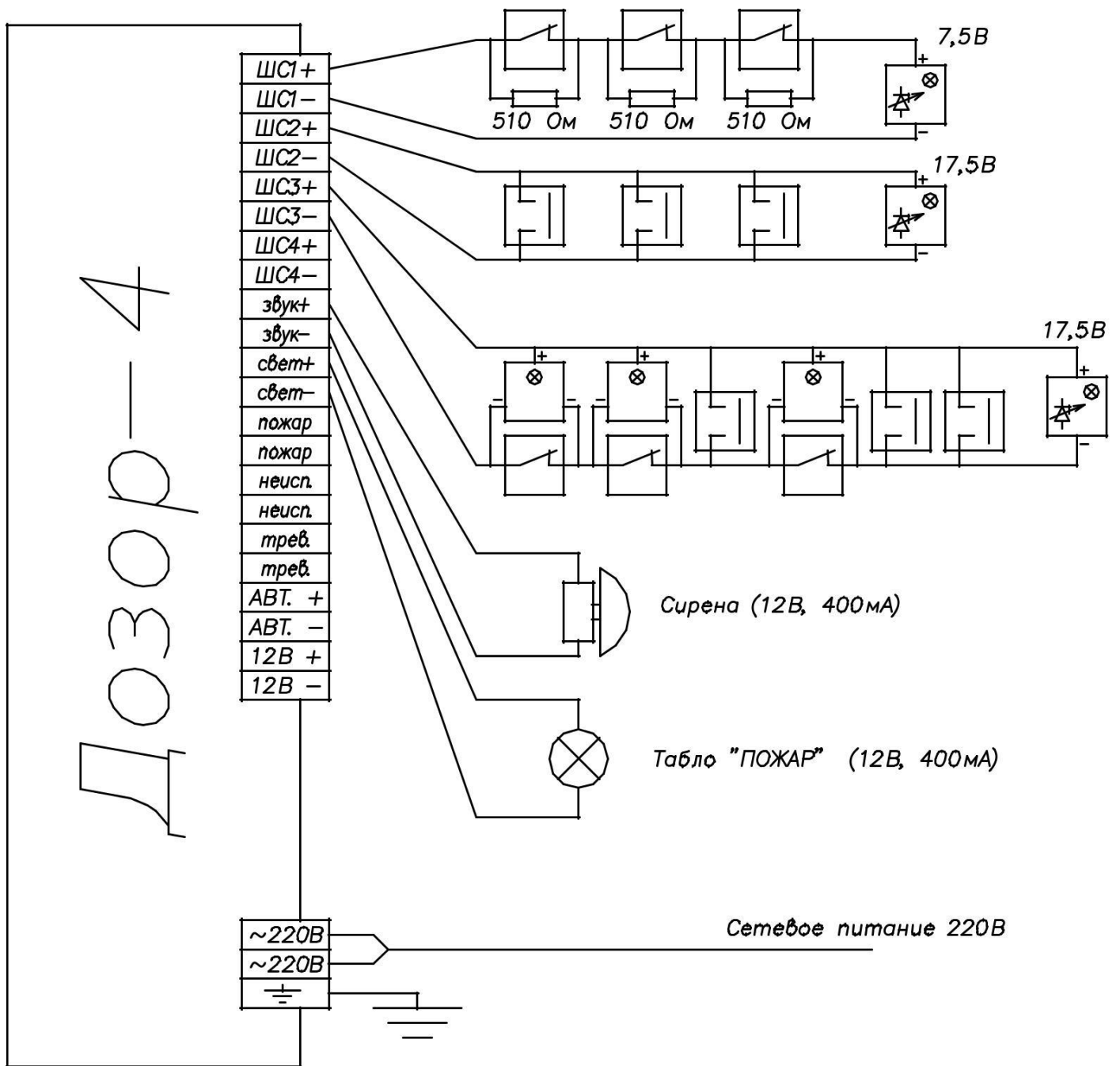
Рисунок 9 - Пример построения пожарной сигнализации на базе прибора ДОЗОР-4
