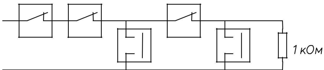
Комбинированный шлейф
