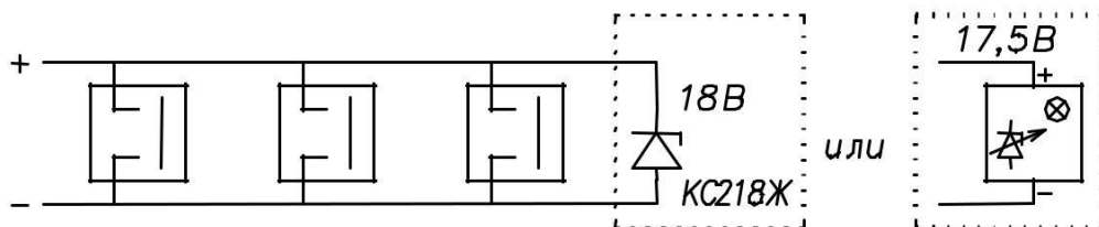
Шлейф с датчиками типа ИГ105
