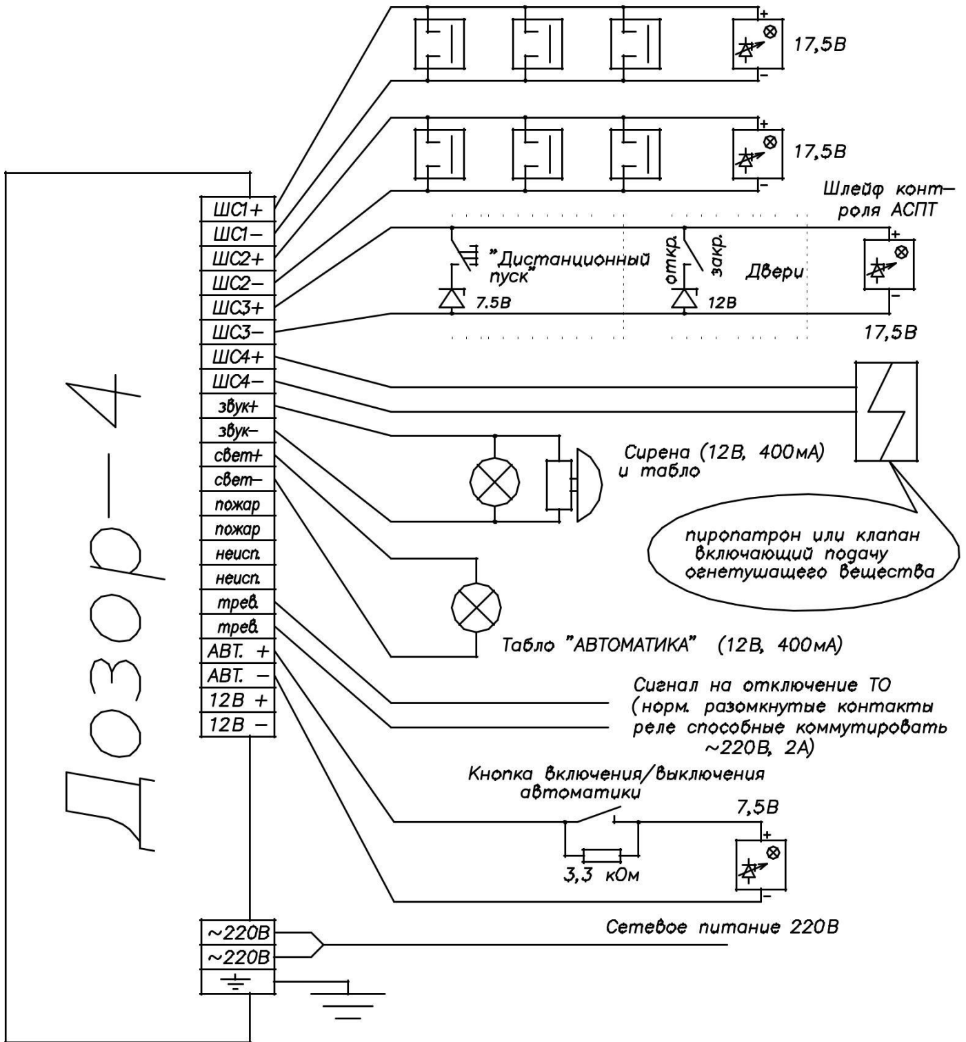
Рисунок 11 - Пример построения автоматической системы пожаротушения на базе прибора ДОЗОР-4
