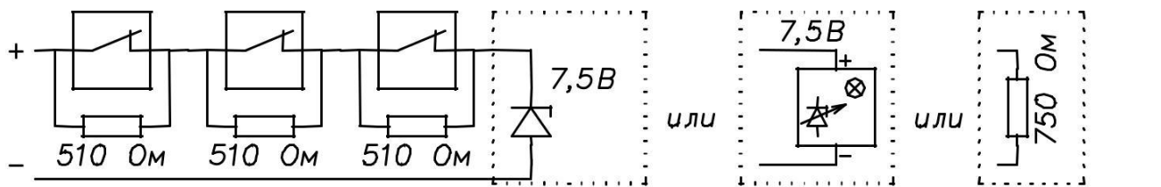
Шлейф с датчиками типа ИГ105
