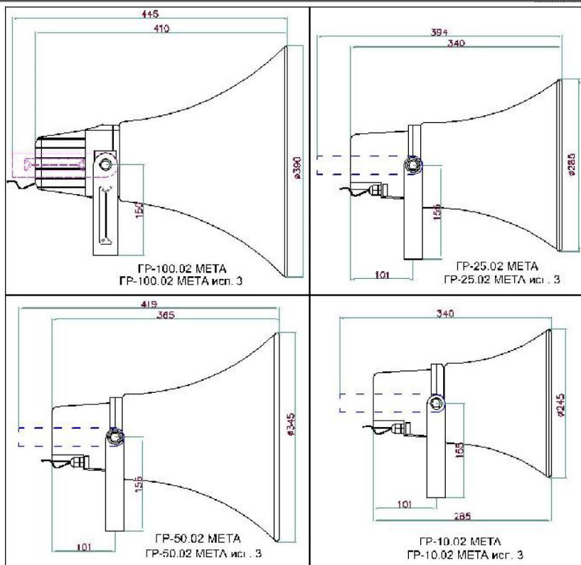
Рис.1. Размеры рупорных громкоговорителей
