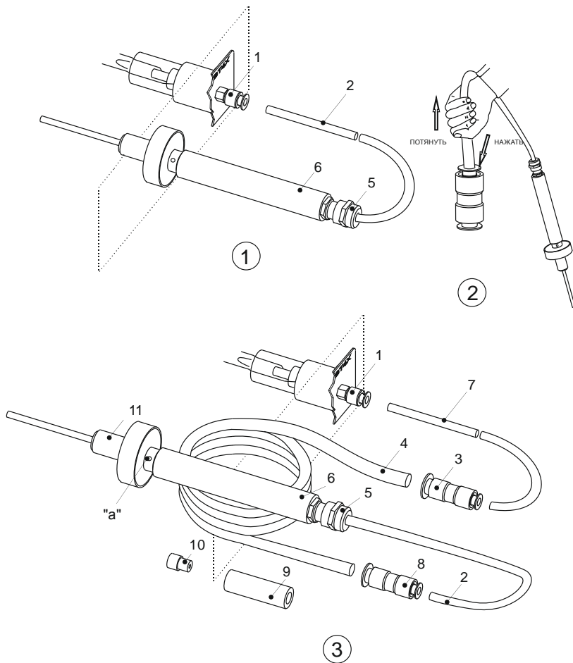
Рис. 3. Схема соединения элементов пробоотборника с газоанализатором (1) и элементов удлинителя с газоанализатором (2)
