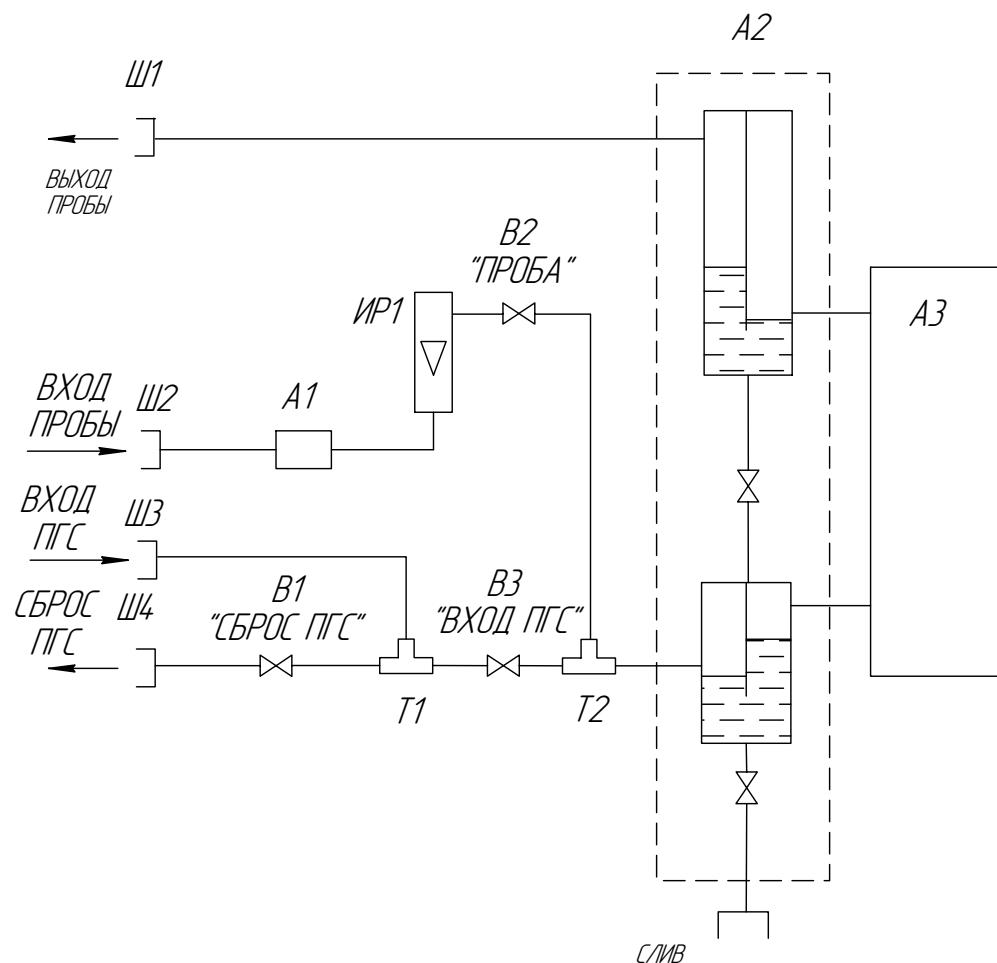
Рисунок 1.2 – Газоанализаторы АНКАТ-500. Схема газовая соединений.
