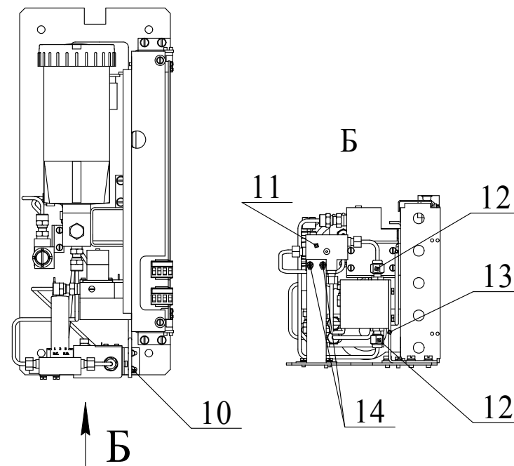
Блок аналитический (извлечен из корпуса поз.1)
