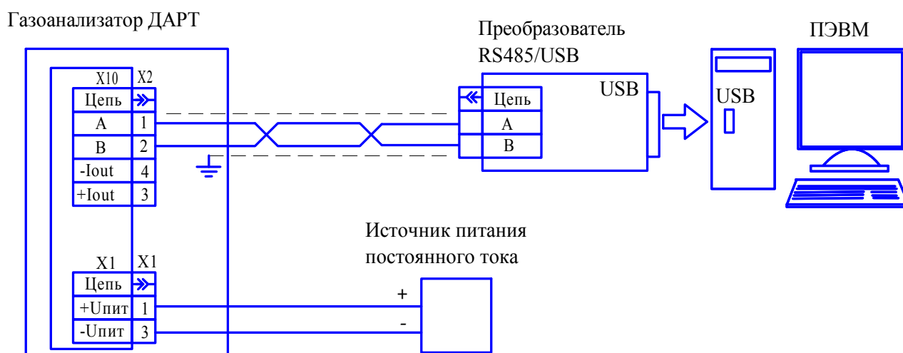
Рисунок 2.3 - Схема подключения газоанализатора к ПЭВМ
