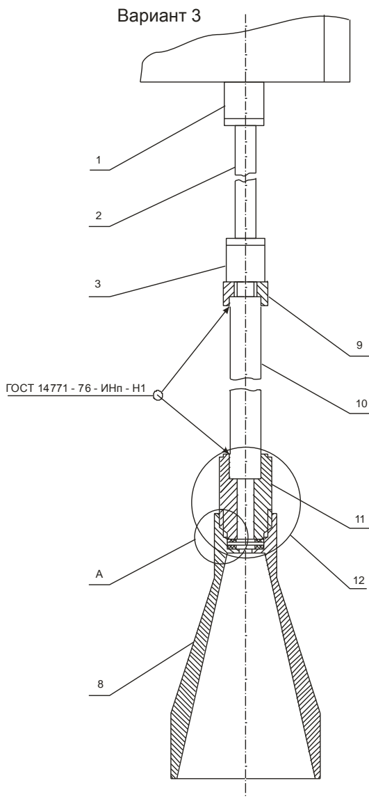
Пробоотборное устройство (вариант 3)
