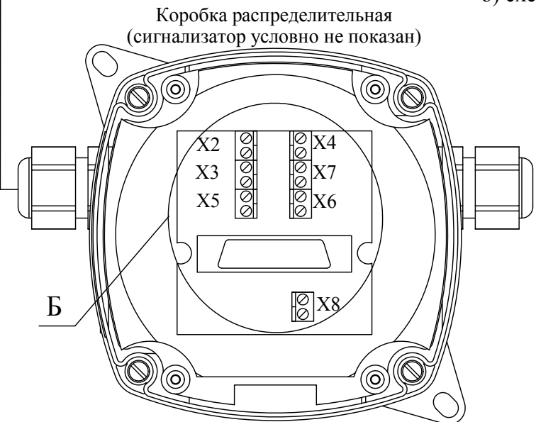
а) сигнализатор СТГ-3 с блоком БПС-3
