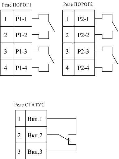
Положение контактов реле в исходном состоянии
