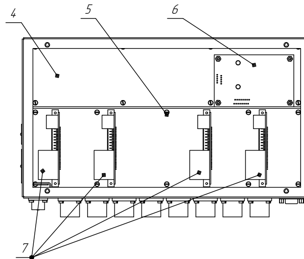
Рисунок 1.1 – Блоки расширения и связи БРС. Внешний вид
